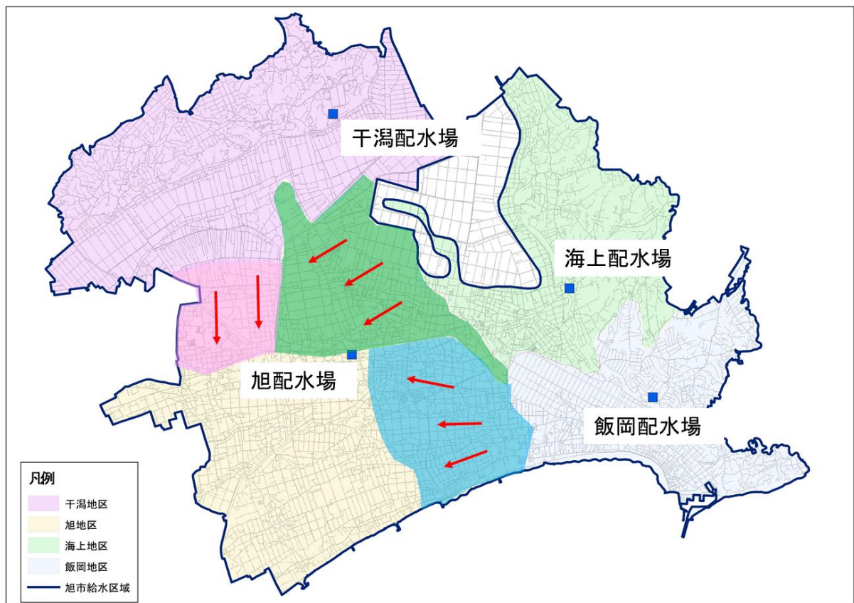
図 5-1 旭配水場の配水区域縮小
