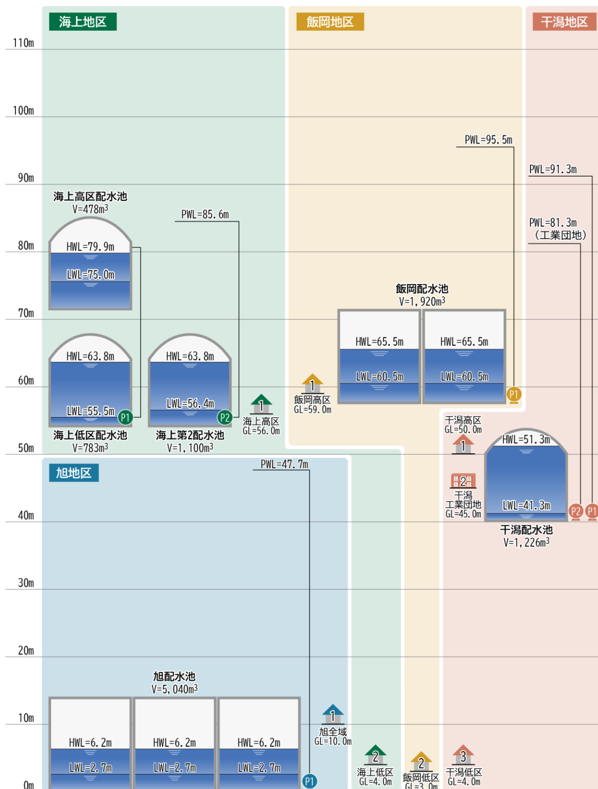
図 2-1 水位高低図
