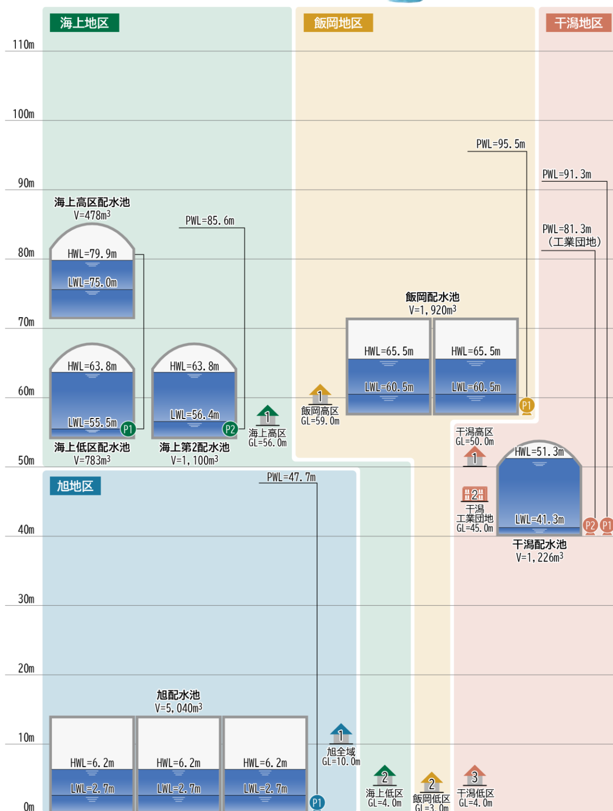
图 2.2.3 水位高低図
