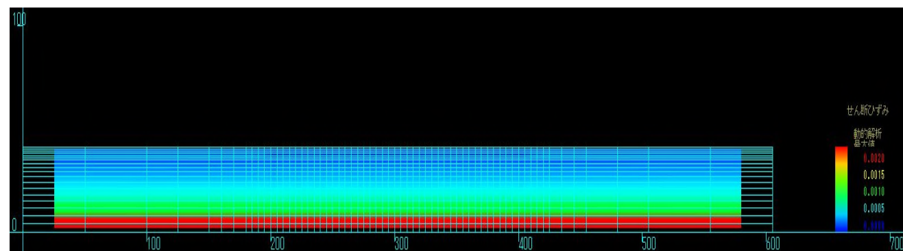
最大せん断方向ひずみコンター図
