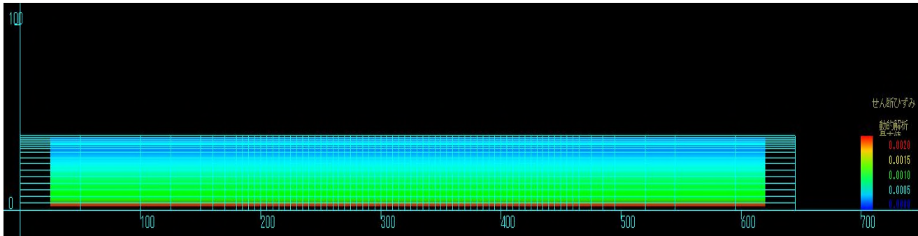
最大せん断方向ひずみコンター図
