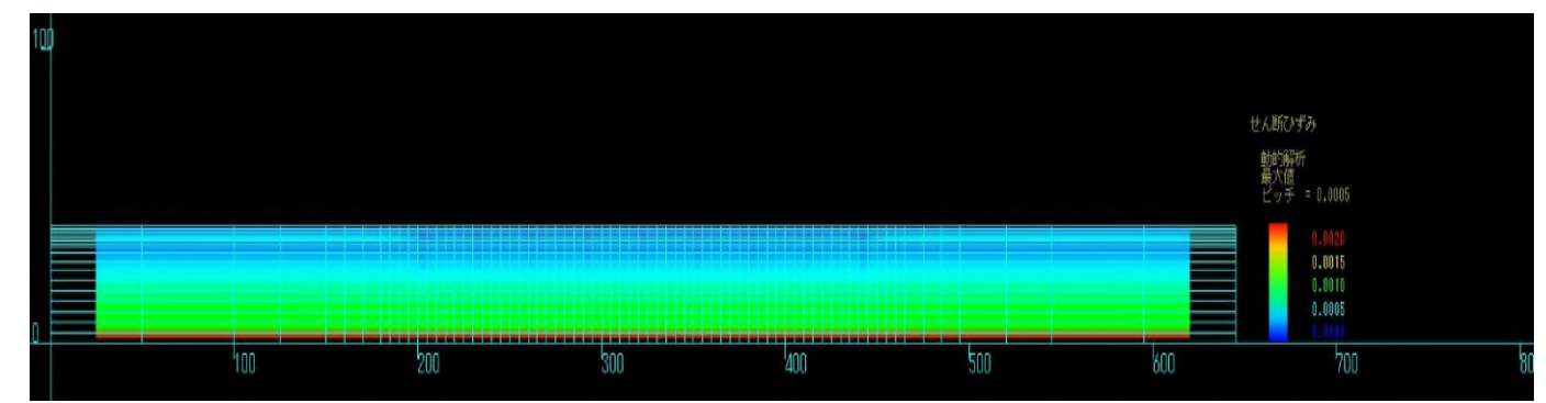
最大せん断方向ひずみコンター図
