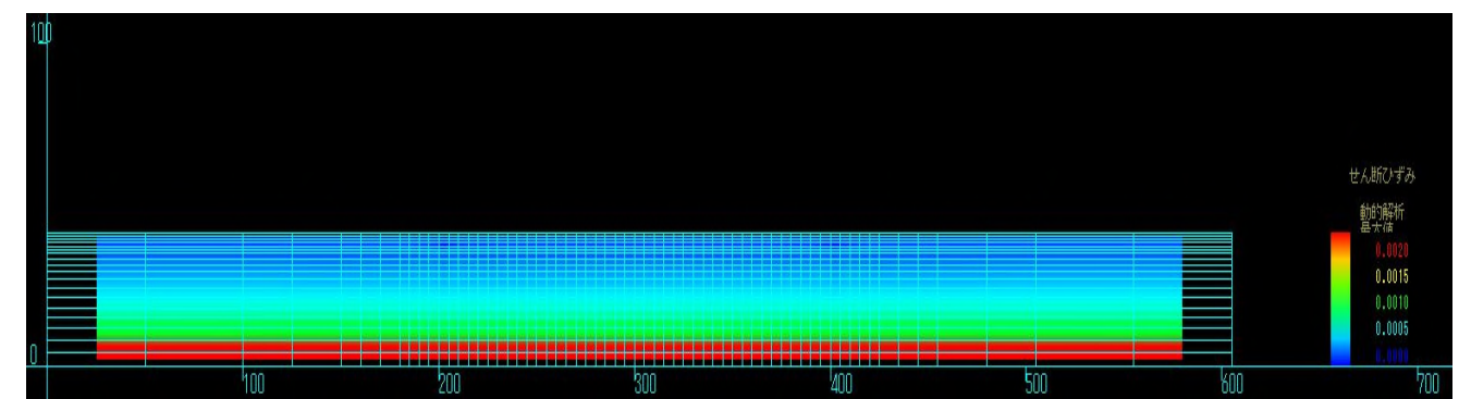
最大せん断方向ひずみコンター図
