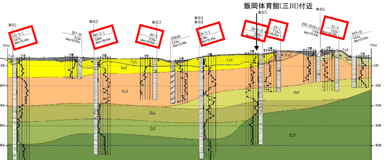
図-5.4 地層断面図(東西 5)
