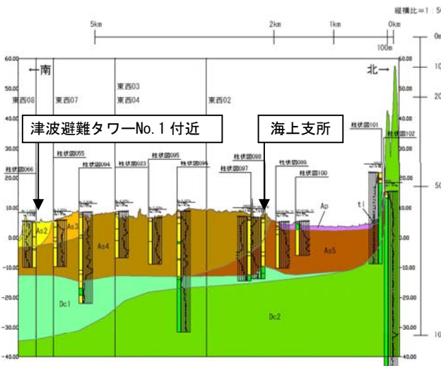
想定地質断面図(南北04)
