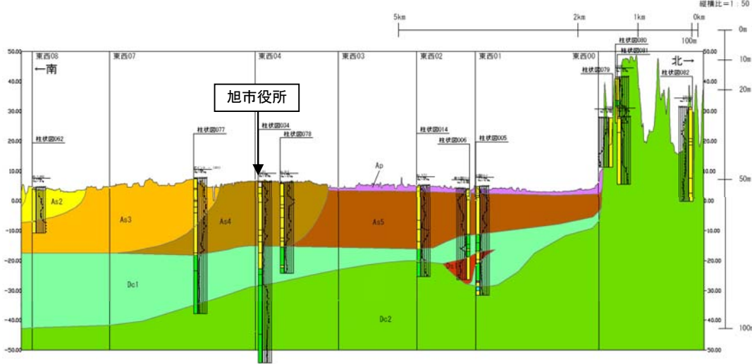
想定地質断面図(南北02)
