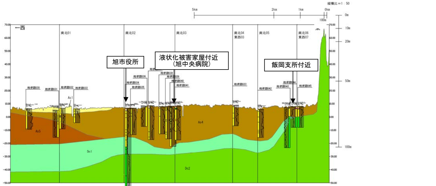
想定地質断面図(東西04)
