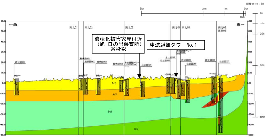
想定地質断面図(東西08)
