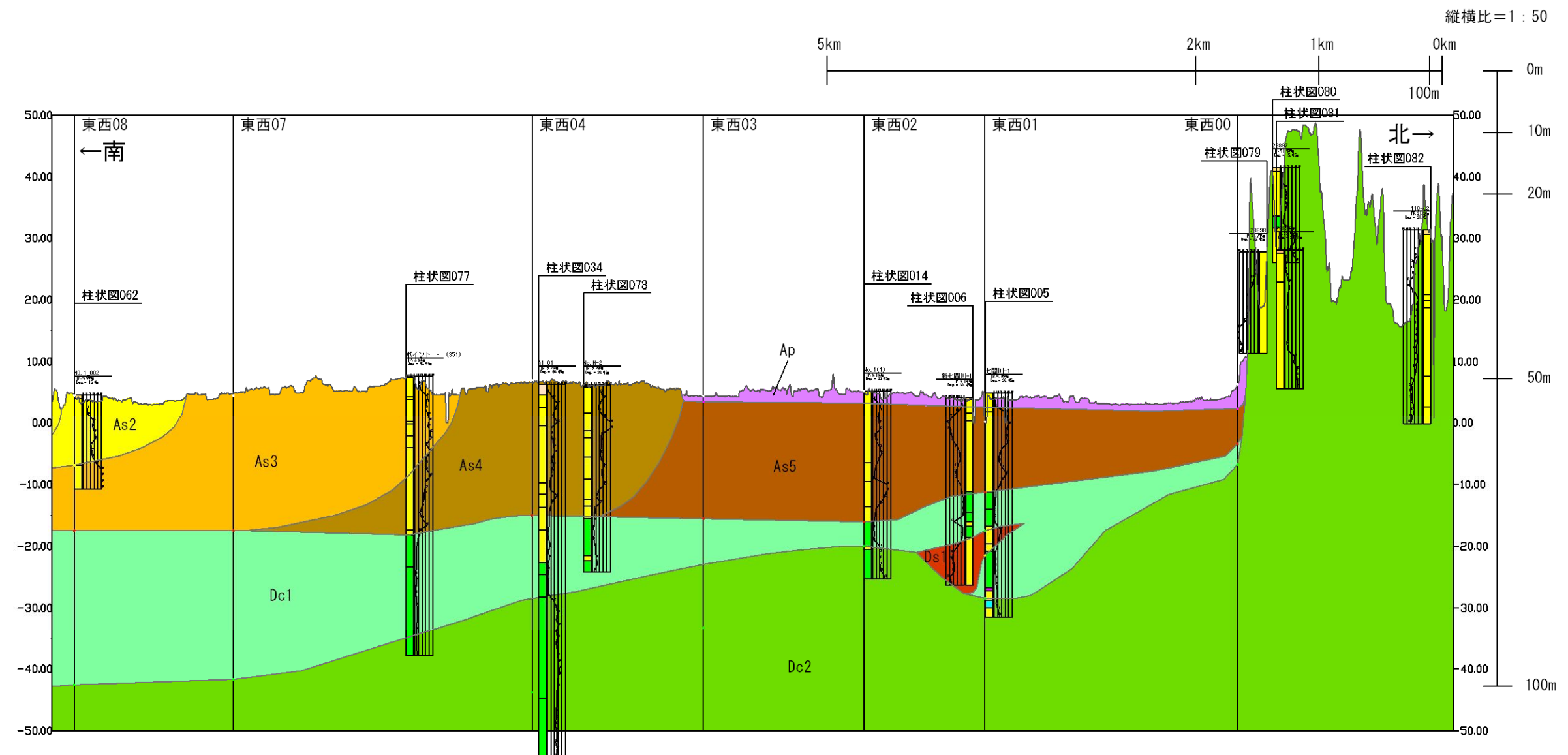
想定地質断面図(南北02)
