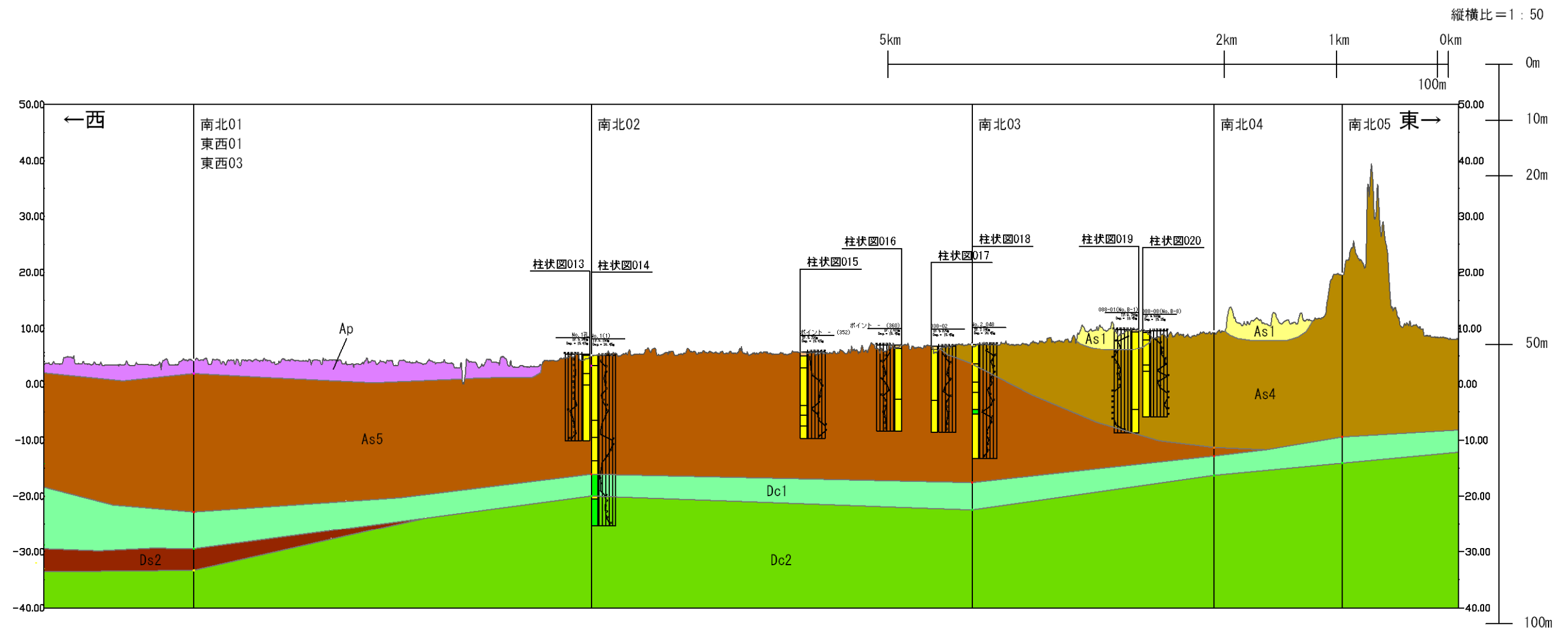
想定地質断面図(東西02)
