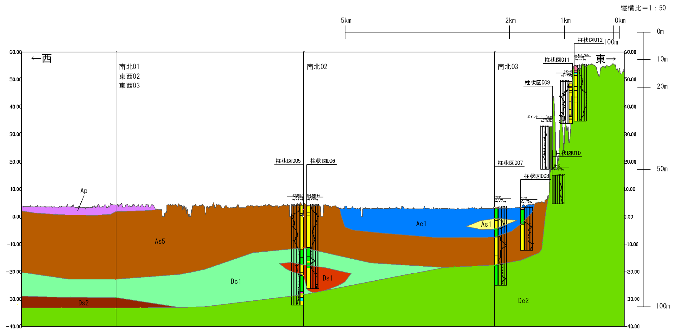
想定地質断面図(東西01)
