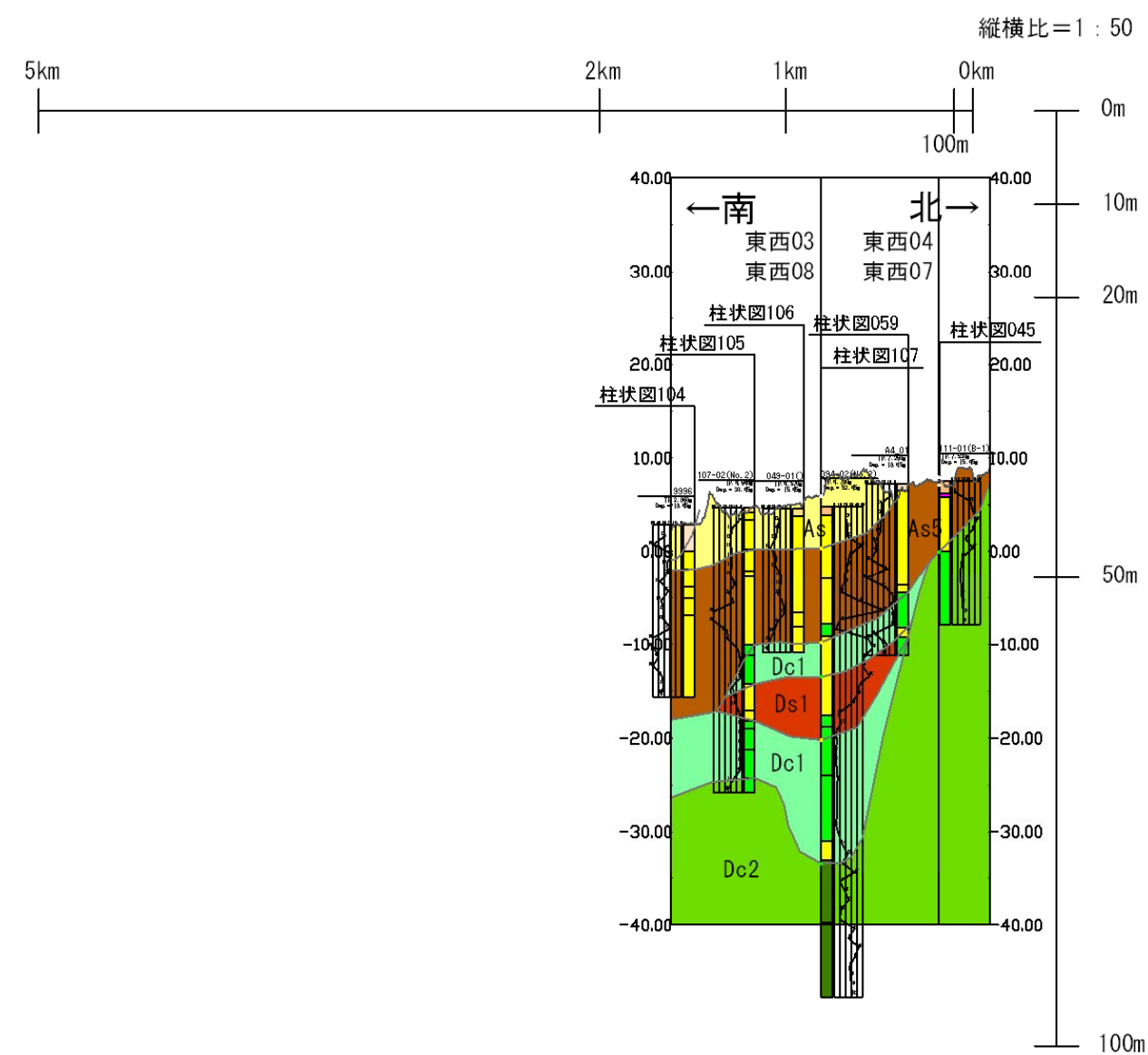
想定地質断面図(南北06)
