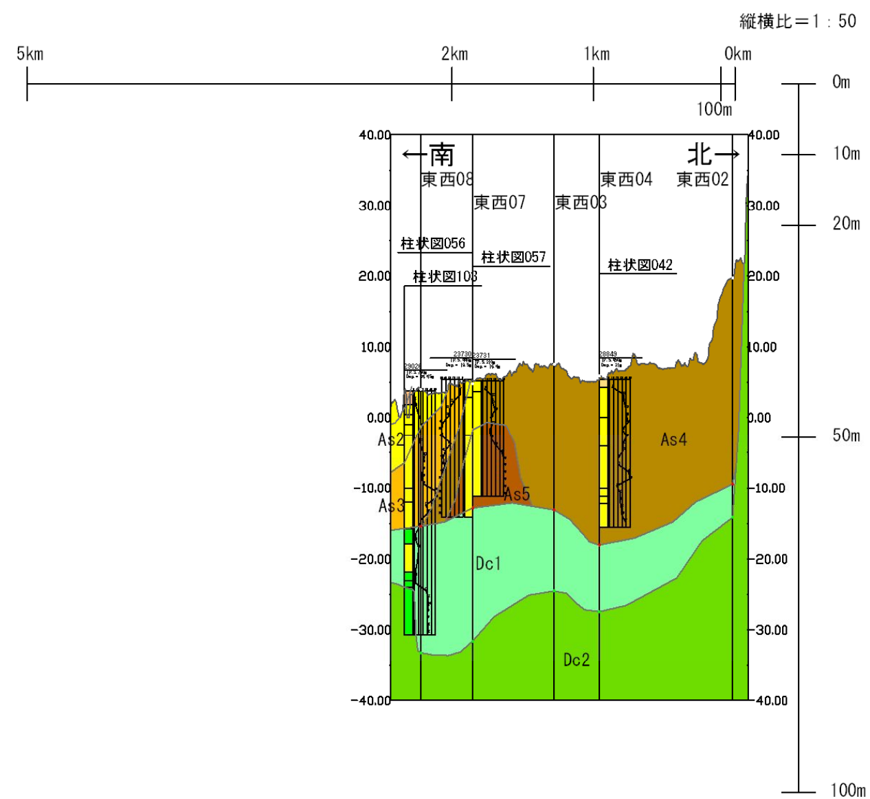
想定地質断面図(南北05)
