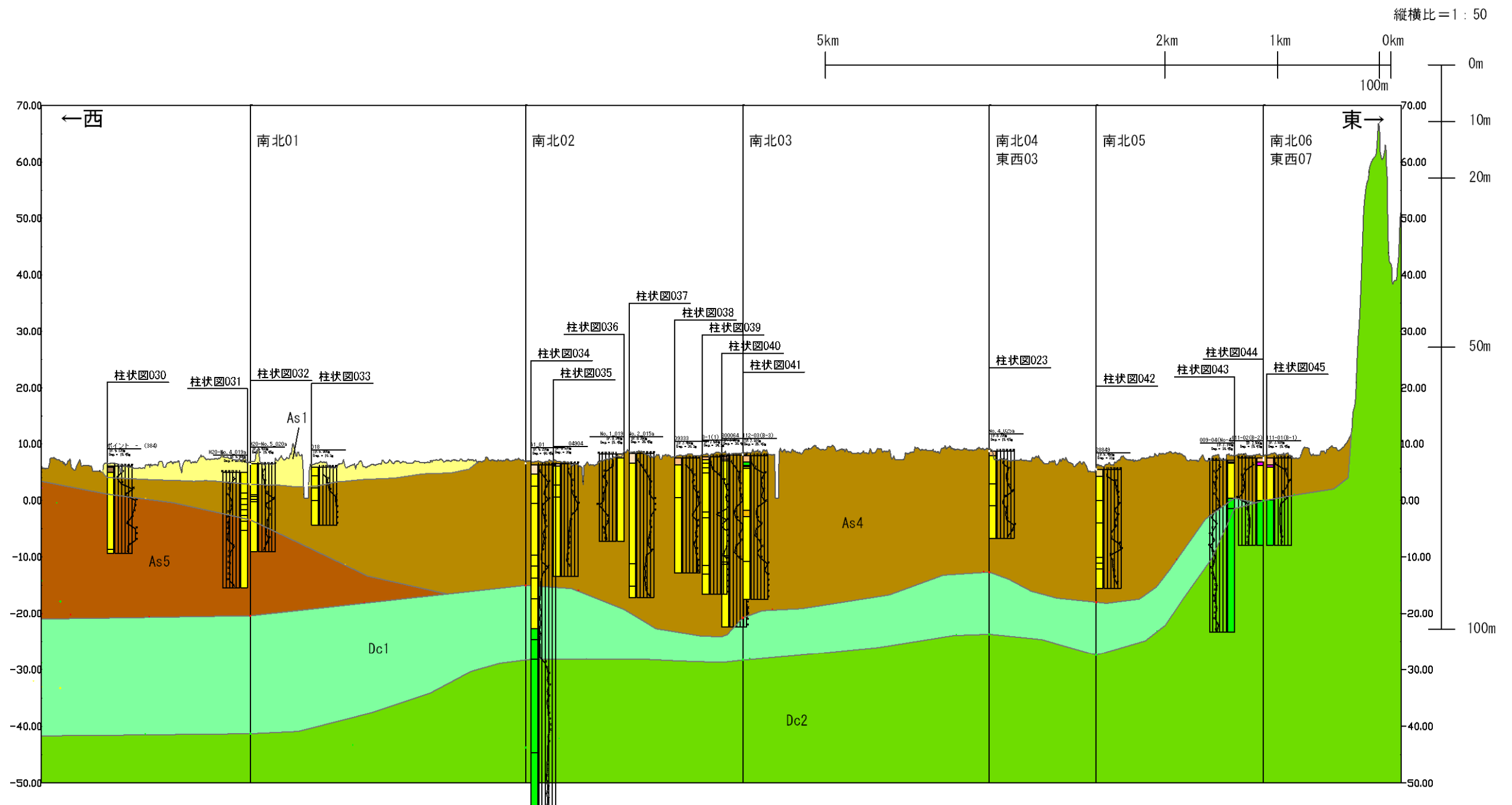
想定地質断面図(東西04)
