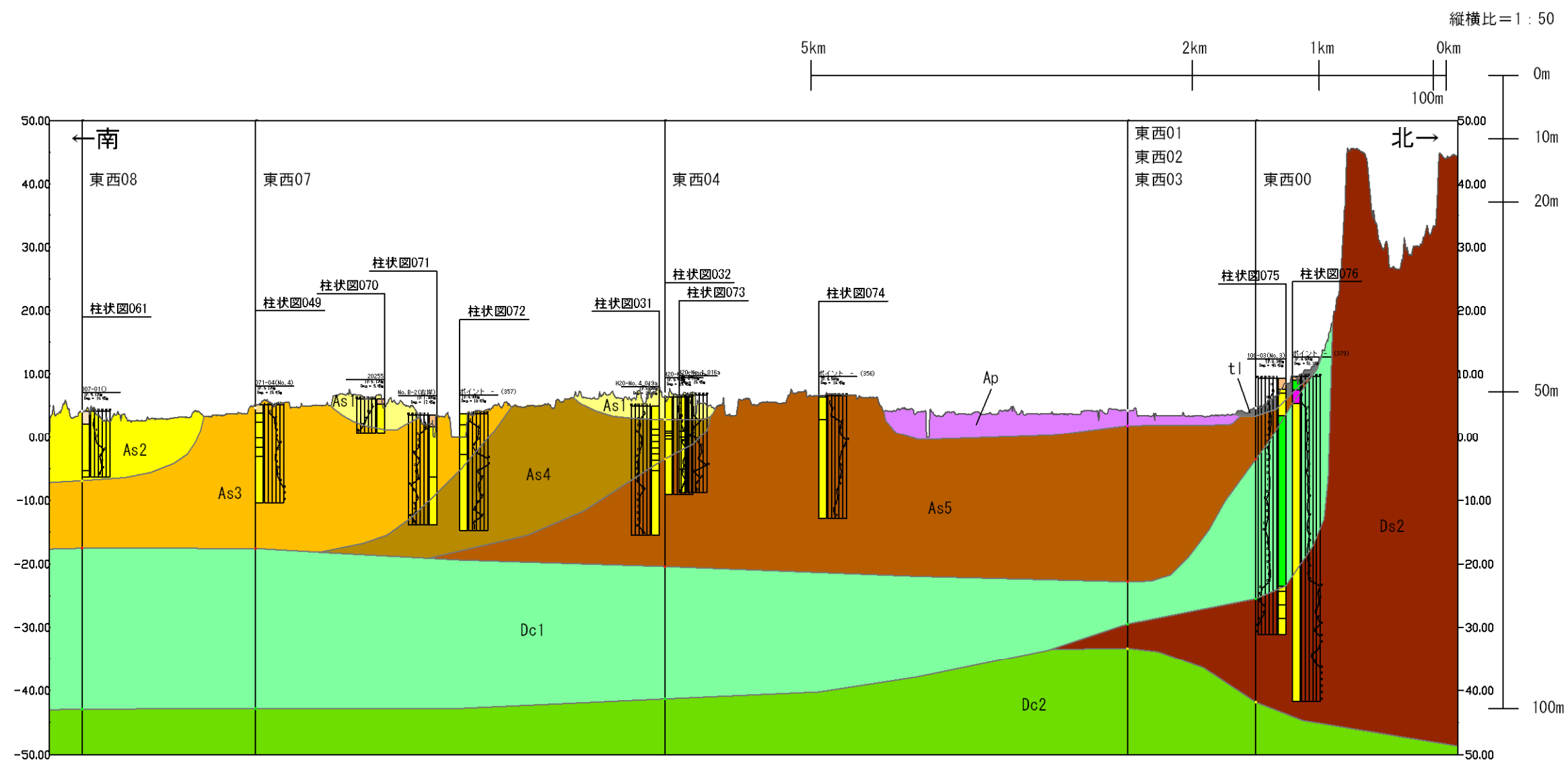
想定地質断面図(南北01)
