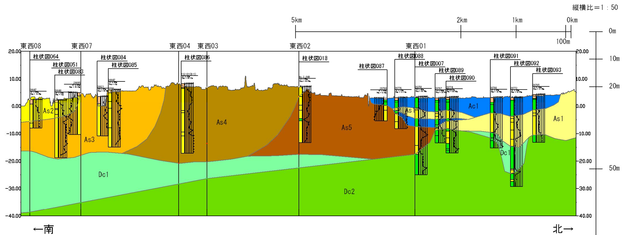
想定地質断面図(南北03)
