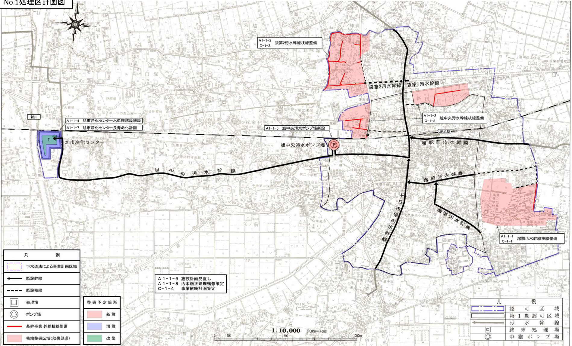
No.1処理区計画図
