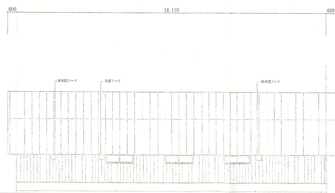
北側立面図
