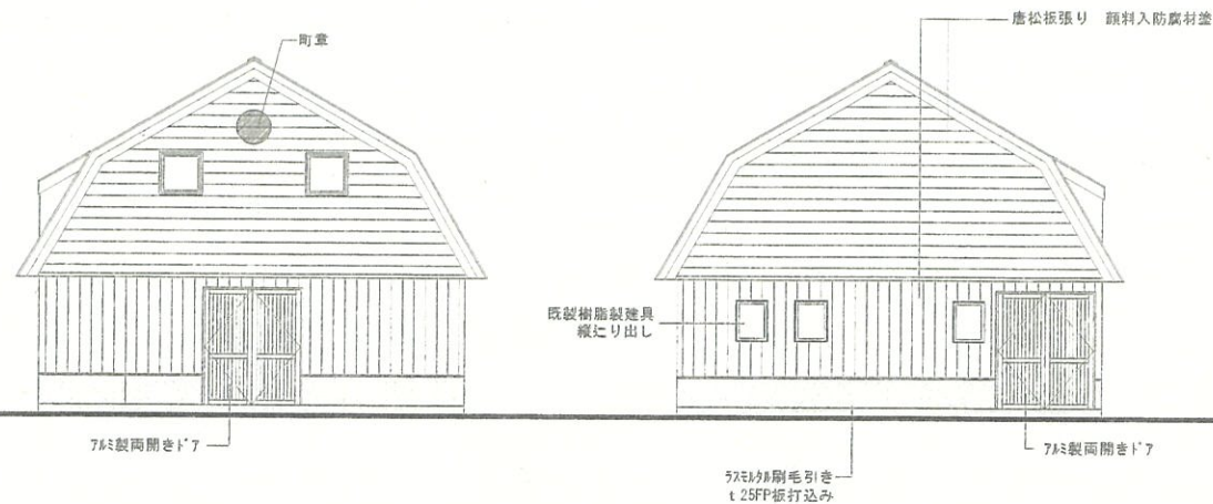
東側立面図
