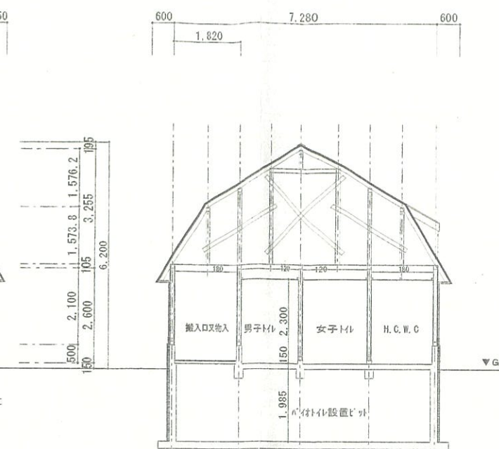
断面図
