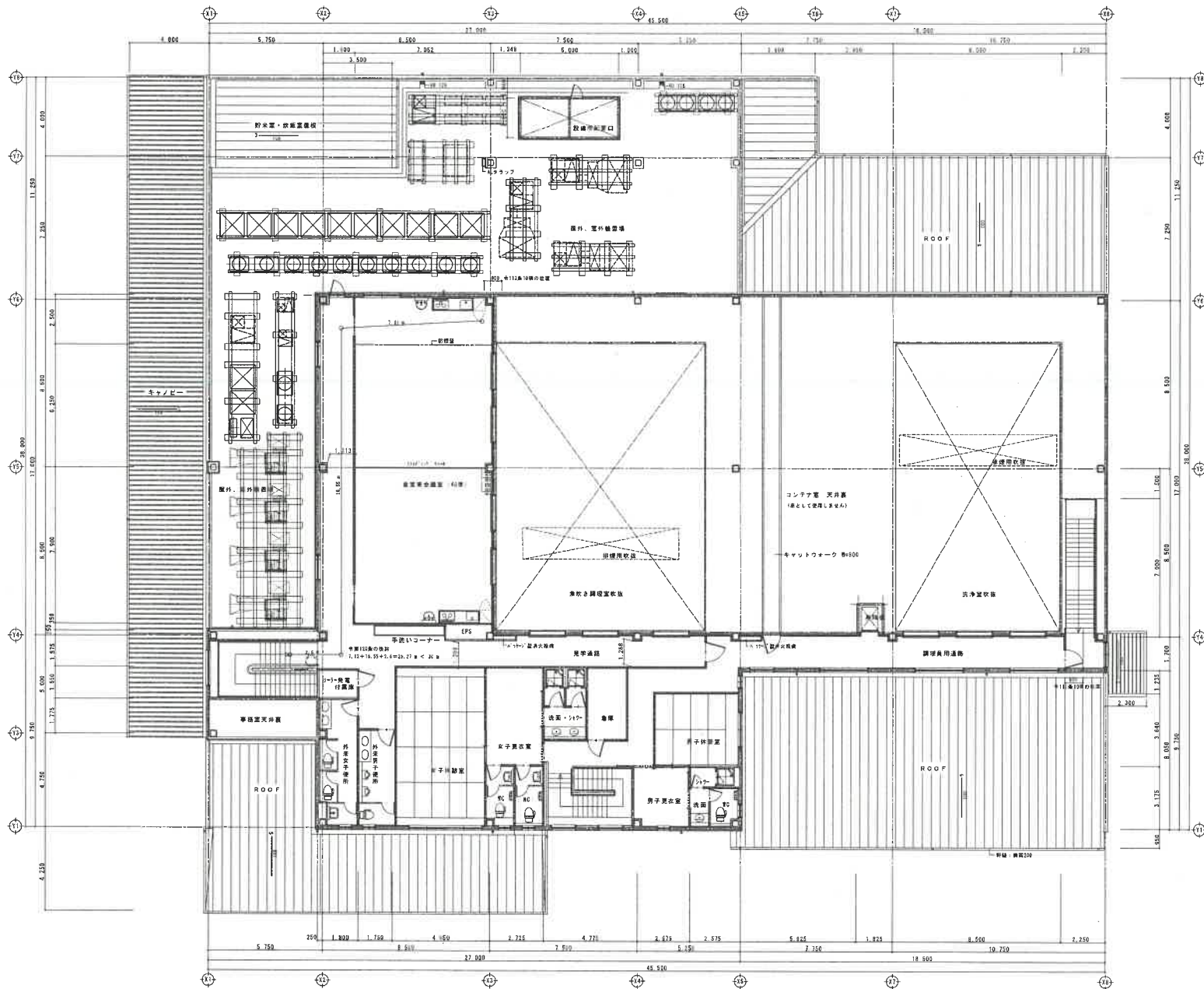
2階平面図 s 1 : 100
