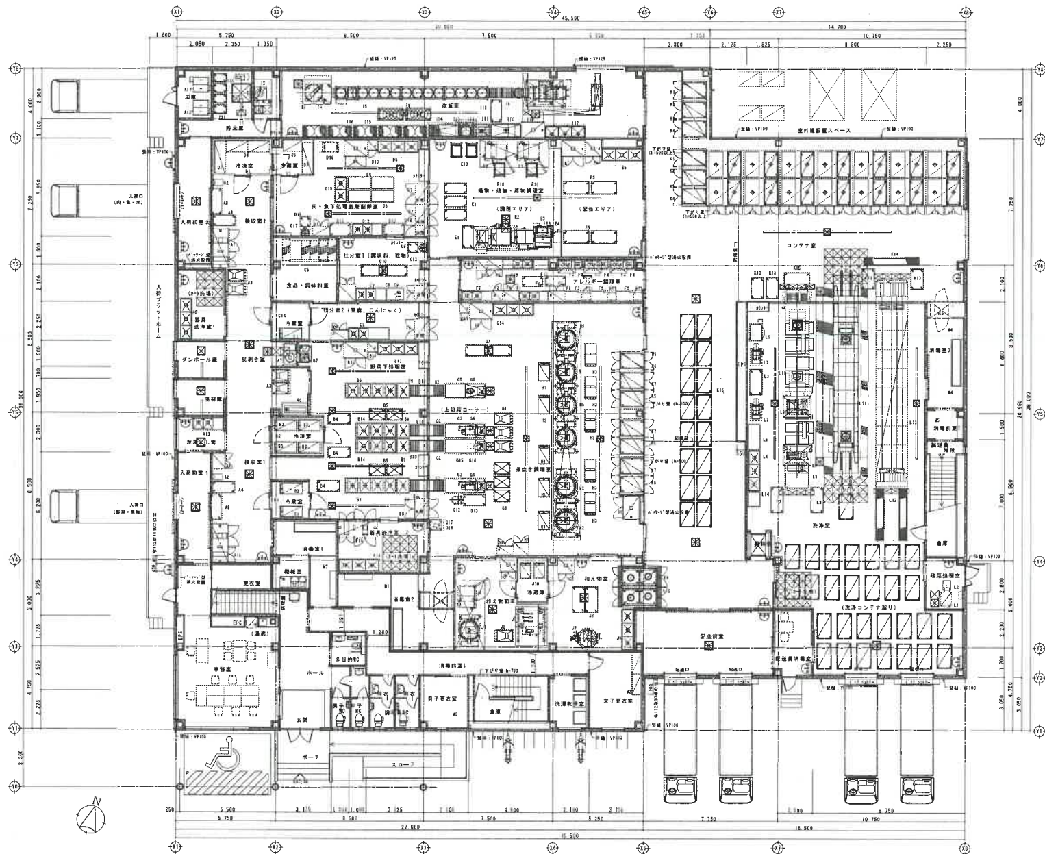
1階平面図 1:100
